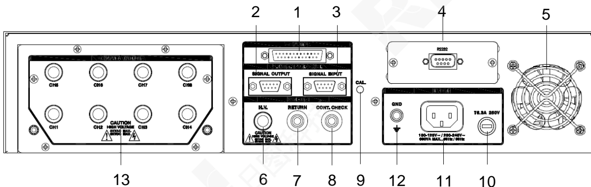
SE 7430 背板说明
