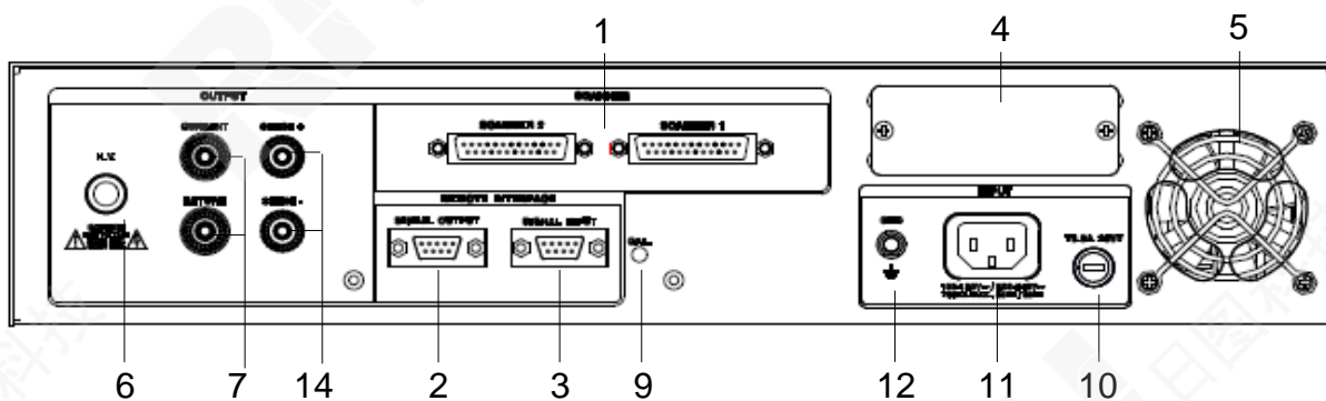
SE 7451 背板说明
